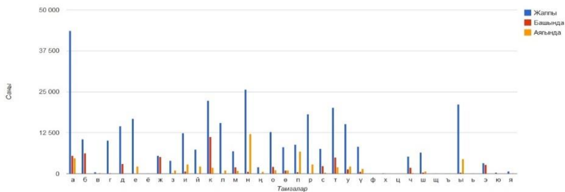
График 9. Мисмилдирик (Бедел белиндеги каргыш) романынын текст ичиндеги тамгалардын сандык статистикасы
