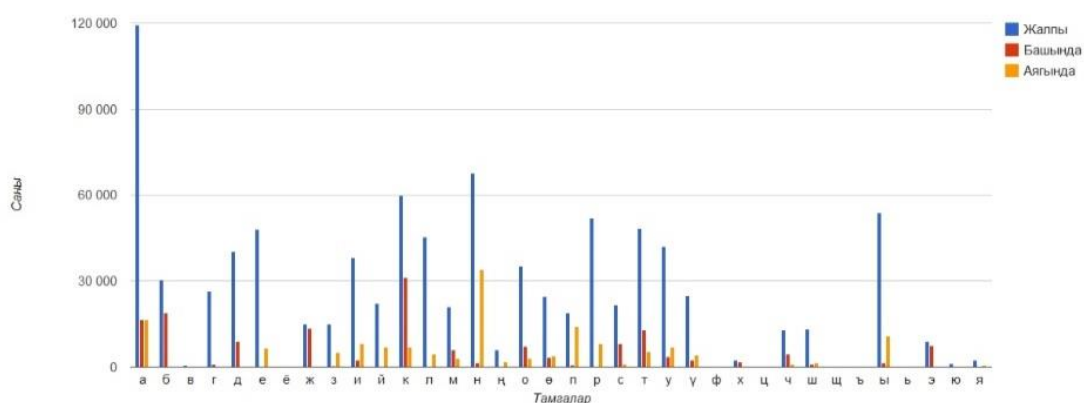
График 17. Хан Ормон романынын текст ичиндеги тамгалардын сандык статистикасы
