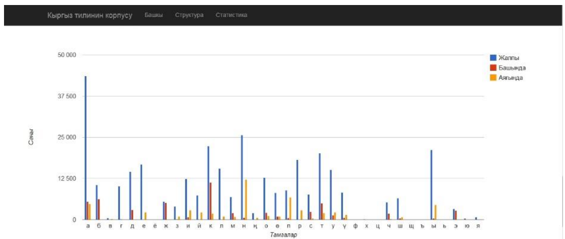
Сүрөт 7. Статистиканын натйжасында түзүлгөн график
