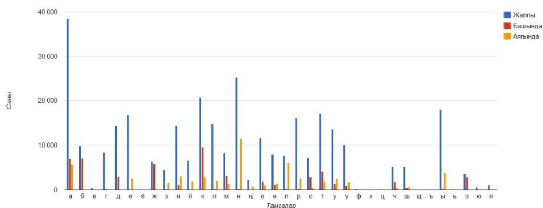
График 11. Өмүр кызык романынын текст ичиндеги тамгалардын сандык статистикасы
