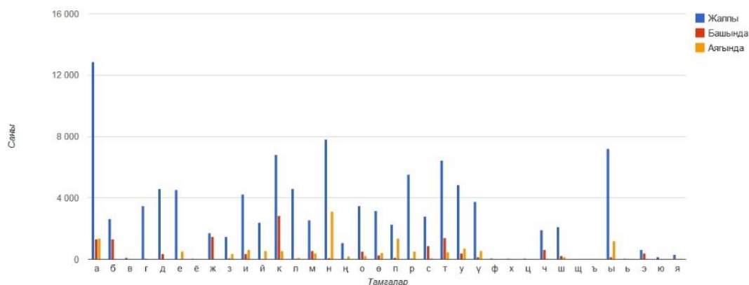
График 12. Өмүр кызык романынын сөздүк ичиндеги тамгалардын сандык статистикасы
