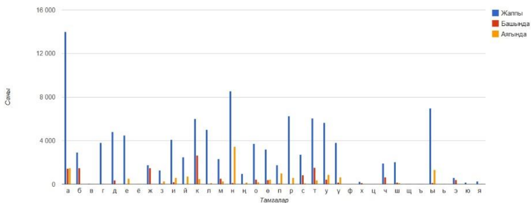
График 6. Барто Чөнө романынын сөздүгү ичиндеги тамгалардын сандык статистикасы
