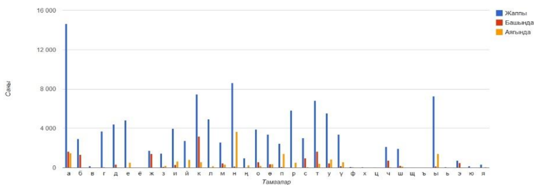
График 2. Айта бар менин кебимди... романынын сөздүк ичиндеги тамгалардын сандык статистикасы
