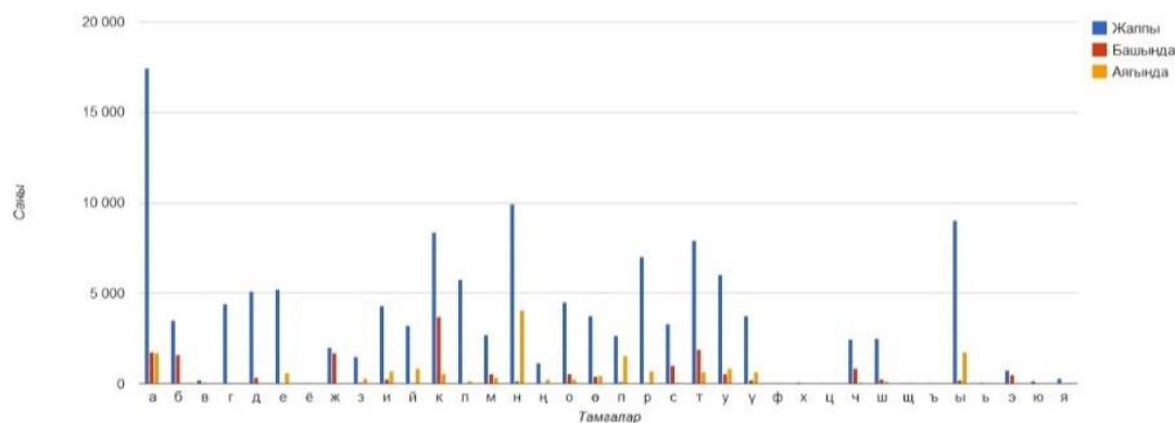
График 10. Мисмилдирик (Бедел белиндеги каргыш) романынын сөздүк ичиндеги тамгалардын сандык статистикасы
