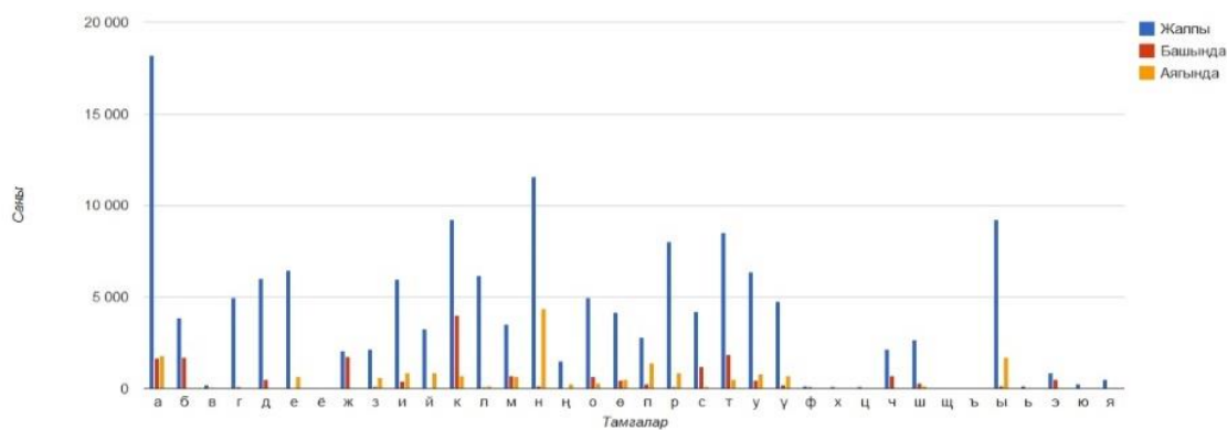
График 4. Башы жок чабендес романынын сөздүк ичиндеги тамгалардын сандык статистикасы
