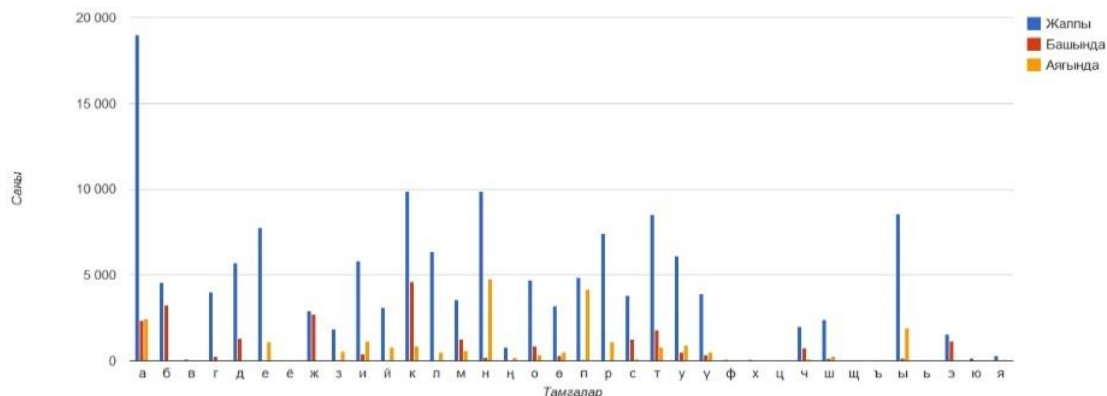
График 15. Улуттун жоголгон байлыгы романынын текст ичиндеги тамгалардын сандык статистикасы
