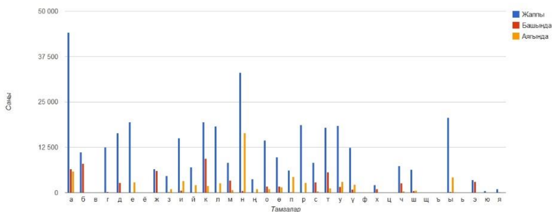
График 5. Барто Чөнө романынын текст ичиндеги тамгалардын сандык статистикасы
