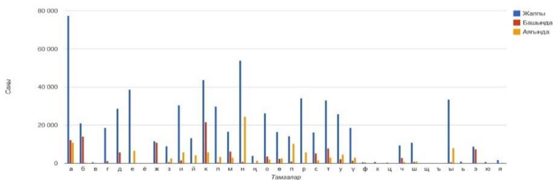
График 3. Башы жок чабендес романынын текст ичиндеги тамгалардын сандык статистикасы
