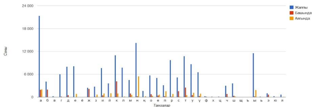
График 8. Мартин Иден романынын сөздүк ичиндеги тамгалардын сандык статистикасы
