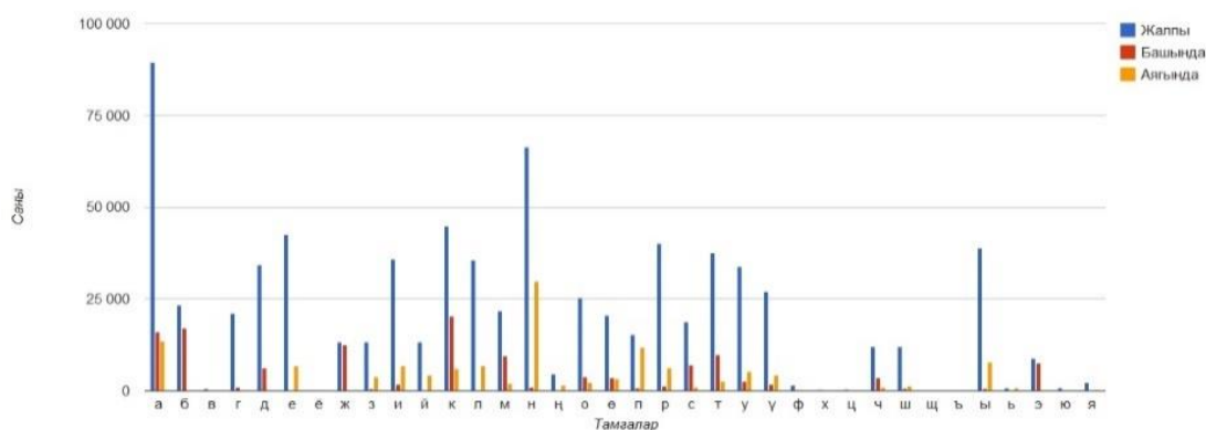
График 7. Мартин Иден романынын текст ичиндеги тамгалардын сандык статистикасы
