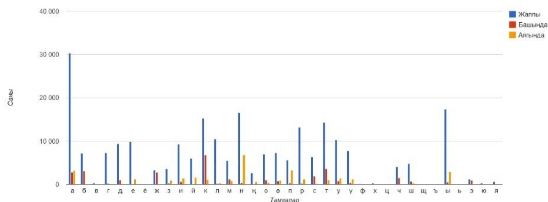
График 14. Сынган кылыч романынын сөздүк ичиндеги тамгалардын сандык статистикасы
