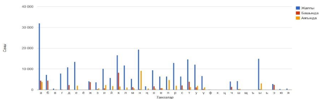
График 1. Айта бар менин кебимди... романынын текст ичиндеги тамгалардын сандык статистикасы
