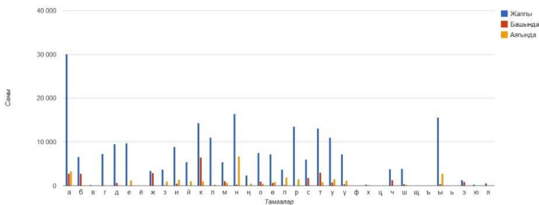
График 18. Хан Ормон романынын сөздүк ичиндеги тамгалардын сандык статистикасы
