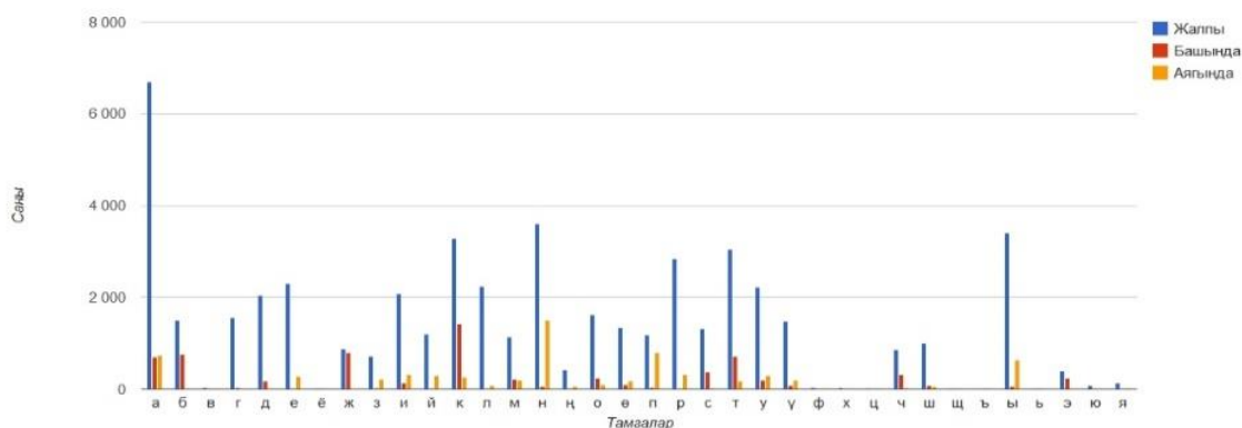
График 16. Улуттун жоголгон байлыгы романынын сөздүк ичиндеги тамгалардын сандык статистикасы
