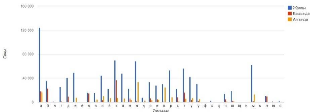
График 13. Сынган кылыч романынын текст ичиндеги тамгалардын сандык статистикасы
